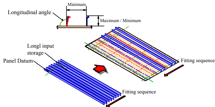
Fig. 3.58. Longitudinal fitting [2]
